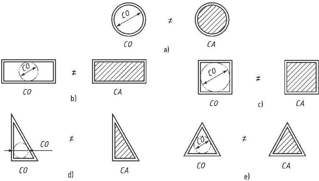
图 D. 3 测定单个井盖或算板有效面积的示意图
