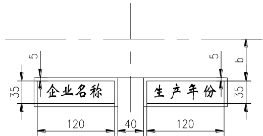
图 F.3 企业名称及生产年份字样位置
