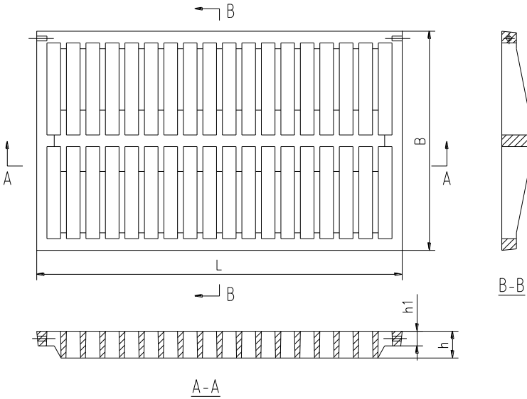
图 E.16 C 级和 D 级 1 型雨水算子结构尺寸示意图
