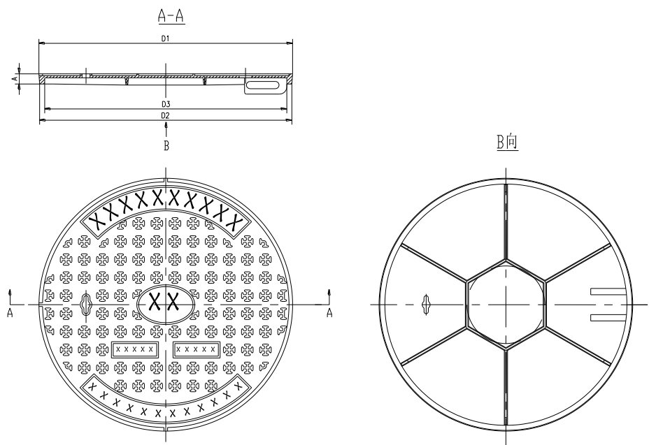
图 E.1 A 级和 B 级井盖结构尺寸示意图
