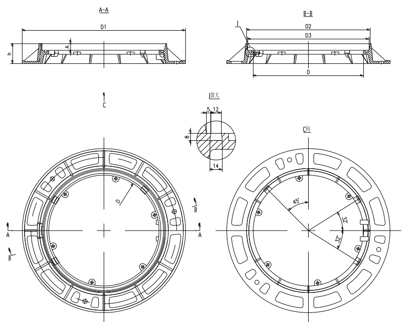
图 E.5 C 级、D 级和 E 级普通井座结构尺寸示意图
