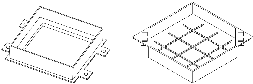
图E.22 适用于给水场合的A级和B级井盖示意图
