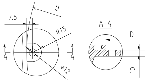
图 E. 7 防坠落网挂耳结构尺寸示意图
