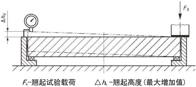
图 A.1 翘起度测量装置示意图
