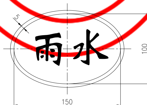
图 F.2 中心字样标识位置及尺寸
