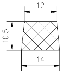
图 E. 15 胶圈横截面
