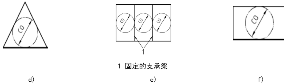
图 3 有效孔径 CO 的示意图
