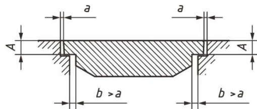
c) 有台阶的井盖/算子(当 b > a 时)
