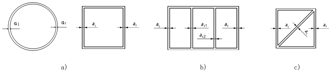
图 2 总间隙示意图
