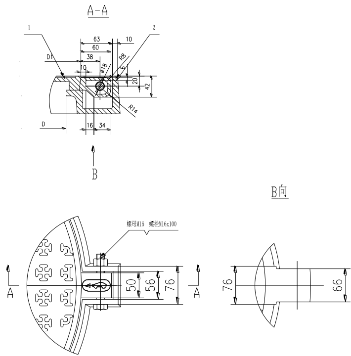
图 E. 28 简易井盖（密封井盖）连接装置
