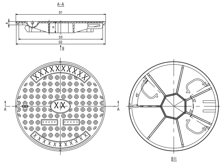
图 E.3 C 级、D 级和 E 级其他井盖结构尺寸示意图
