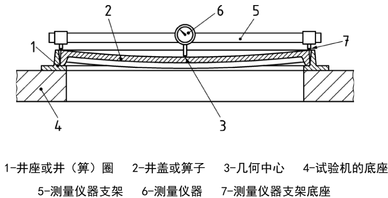
图 B.2 残余变形测量装置示意图
