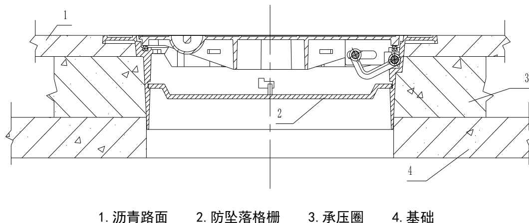
图 G.1 可调式防沉降球墨铸铁井盖的安装示意图
