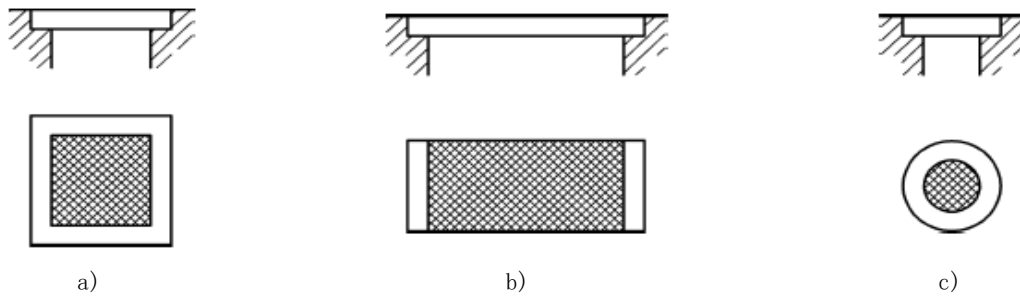
图 4 有效孔径面积的示意图
