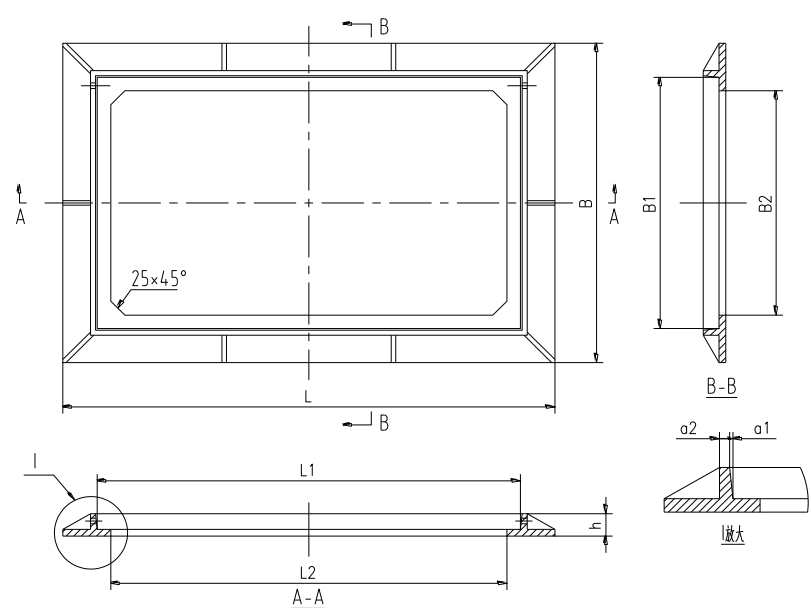
图 E.19 C 级和 D 级井圈结构尺寸示意图
