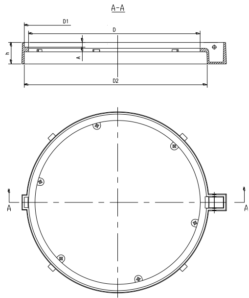
图 E. 25 简易井座结构尺寸示意图
