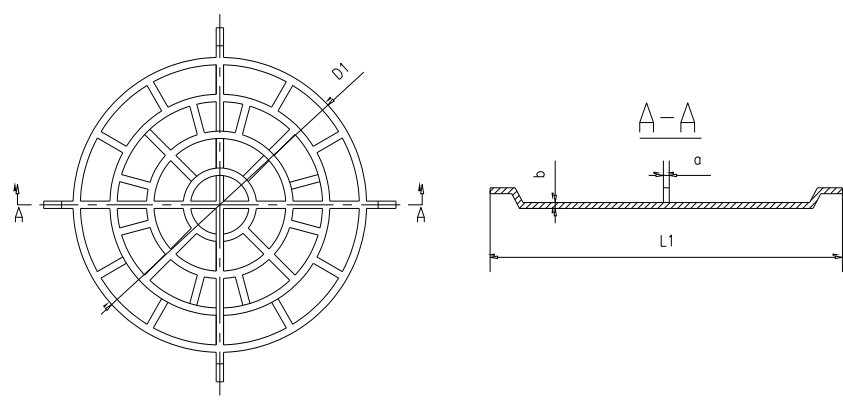
图 E. 8 防坠落格栅结构尺寸示意图
