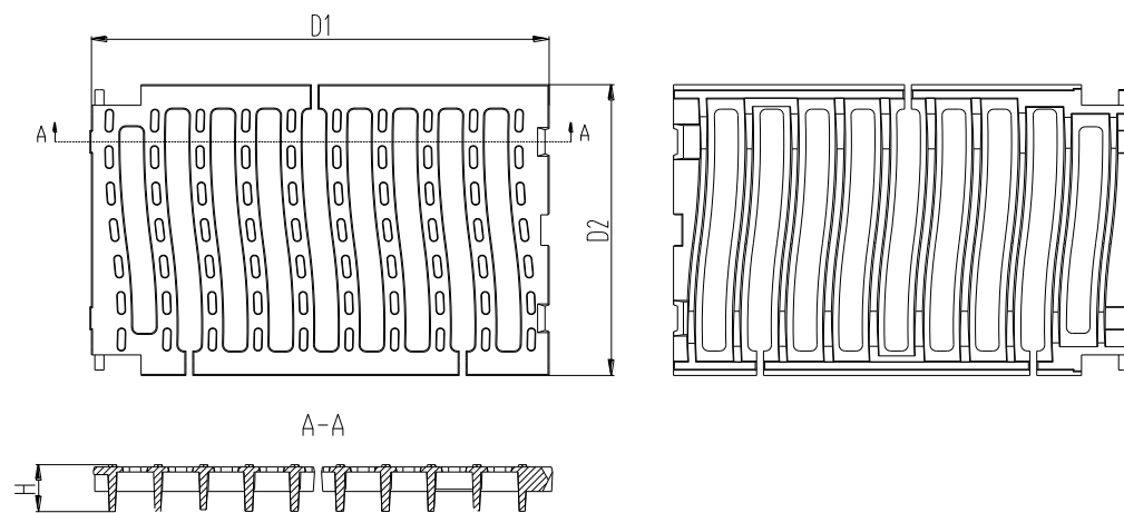
图 E.18 C 级和 D 级可调式防沉降算子结构尺寸示意图
