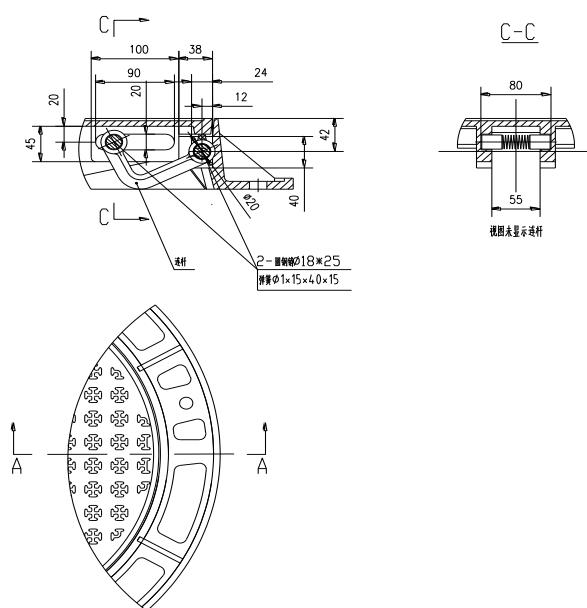
图 E.12 普通井盖连接装置 (暗装铰链)
