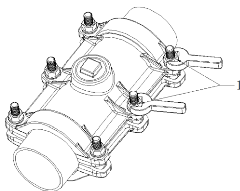
1. 上螺母
